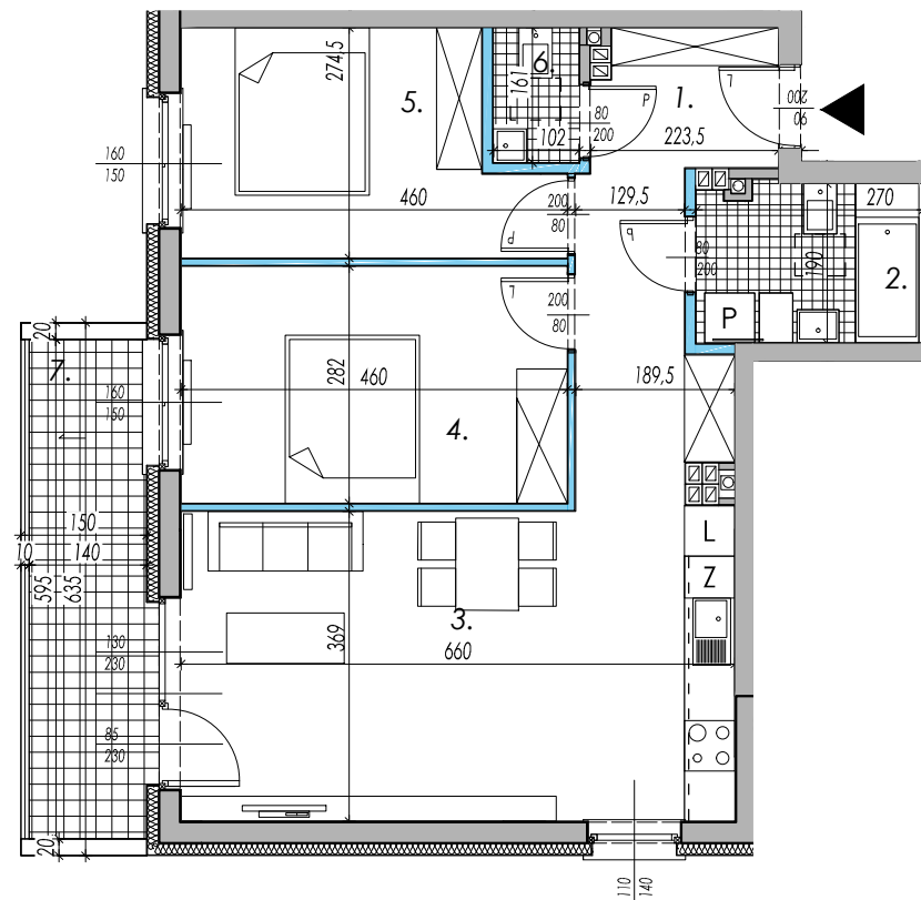
RZUT MIESZKANIA
